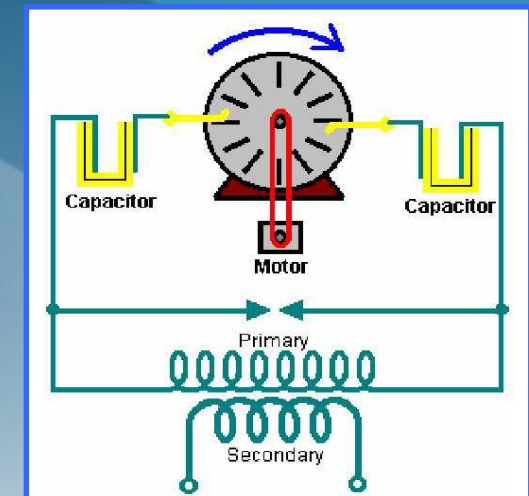
Paul Baumann's Testatica Generator => (équivalent des Figures 1 et 5 de Plauston)
