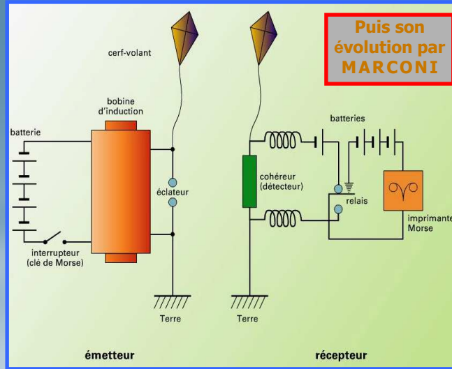
Montage utilisé par Guglielmo Marconi (1874-1937) dans ses premiers essais de télégraphie sans fil (T.S.F.) en 1894. Perfectionnant l'émetteur à étincelles de Hertz et le récepteur (pour lequel il utilise un cohéreur comme détecteur et en leur associant une grande antenne verticale tenue par un cerf-volant), il parvient à une transmission télégraphique sur 2,5 Km
