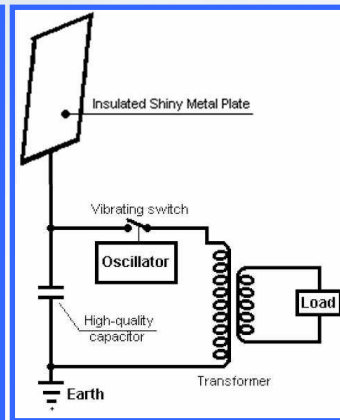
Principe d'émetteur à arc et Récepteur d'Energie Radiante de Nicolas TESLA (1856-1943), sur les traces de HERTZ , MARCONI ...
