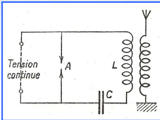
Principe d'émetteur à arc et Récepteur d'Energie Radiante de Nicolas TESLA (1856-1943), sur les traces de HERTZ , MARCONI ...
