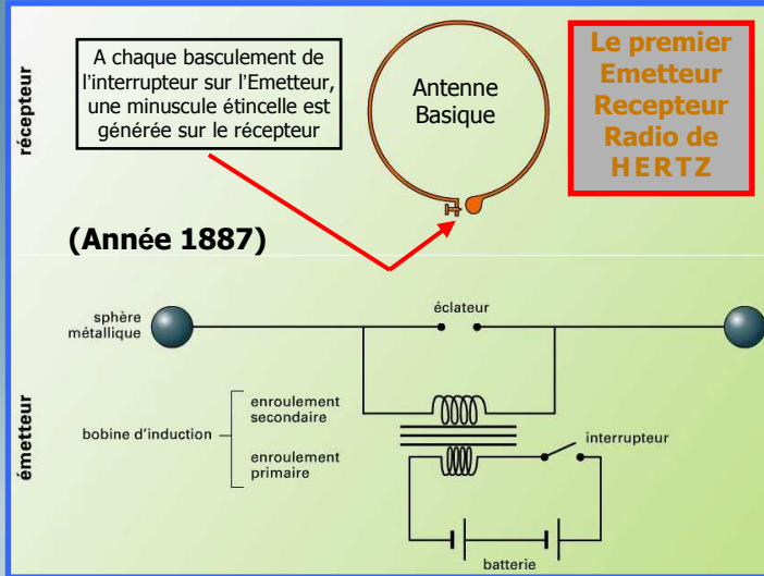
Emetteur / récepteur à arc de Heinrich Hertz (1857-1894), démontrant l'existence des ondes électromagnétiques postulées par James Maxwell en 1864, appelées par la suite " Ondes Hertiennes " en Radio-Communication.
